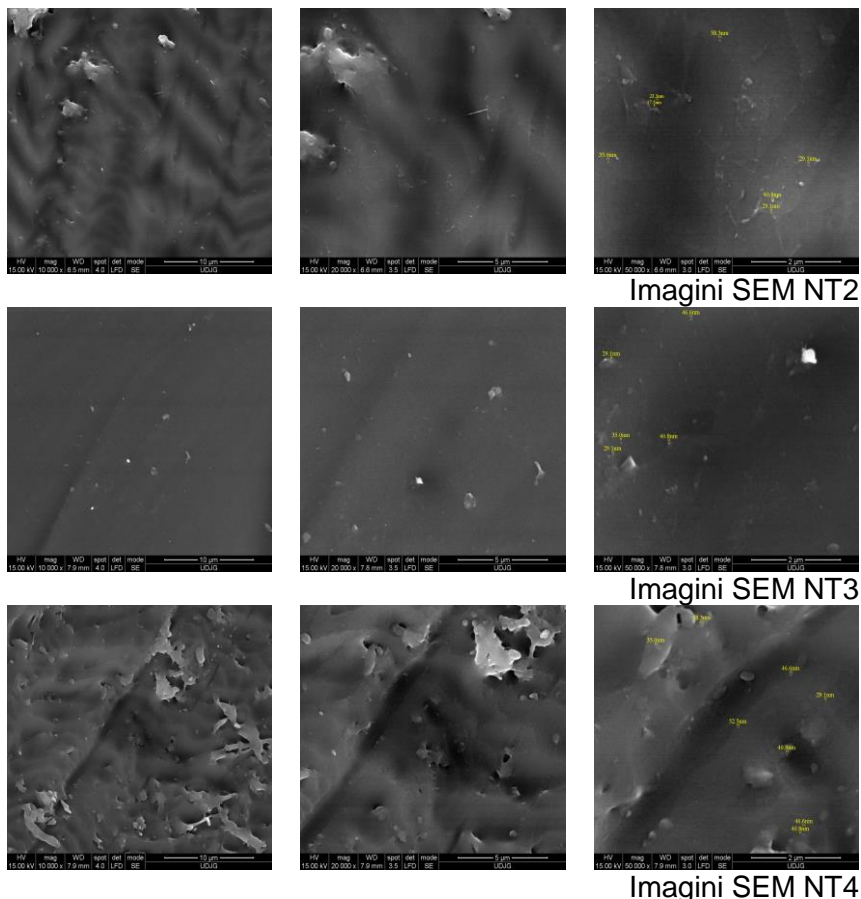
Figura 6. Analiză SEM a materialelor NT
