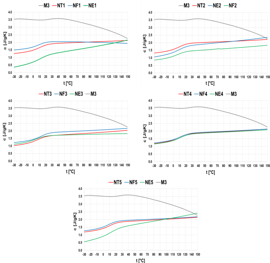
Figura 4. Curbele de variație ale căldurii specifice cu temperatura – durate egale ale tratamentelor
