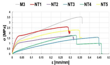
Figura 58. Curbele \sigma/\epsilon pentru materialele NT și comparația comportamentelor medii cu comportamentul mediu al M3
