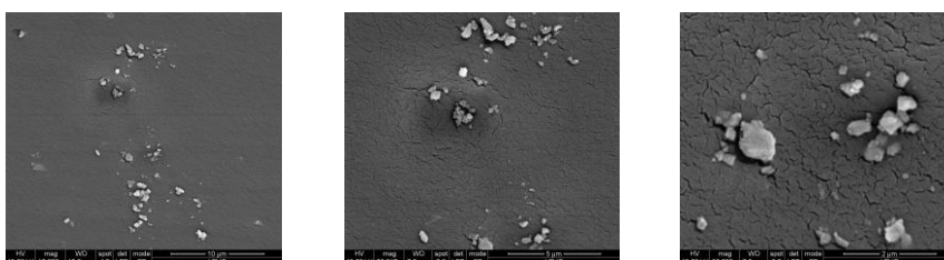
Figura 36. Imagini SEM ale materialului B(g)6 (prima zonă de investigare)
