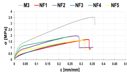
Figura 1. Curbele efort-deformație – materialele NF
