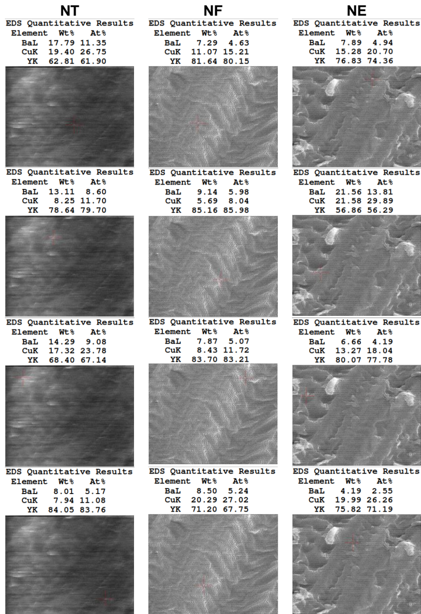
Fig. 10 Analize elementale punctuale pentru materialele expuse tratamentelor speciale timp de 72 de ore
