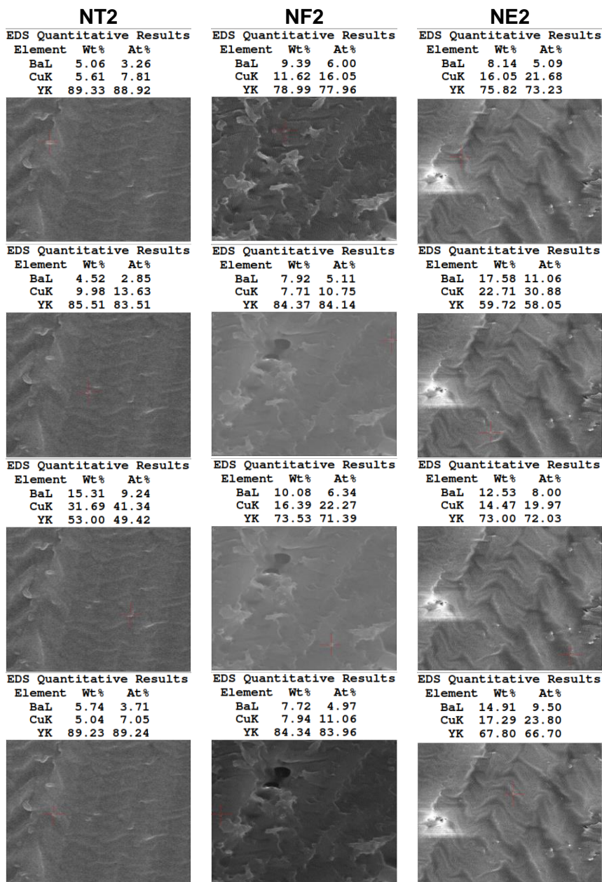
Fig. 9 Analize elementale punctuale pentru materialele expuse tratamentelor speciale timp de 48 de ore
