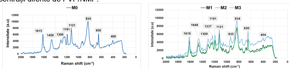
Figura 13. Spectrele Raman ale materialelor modificate (comparație cu M0)
