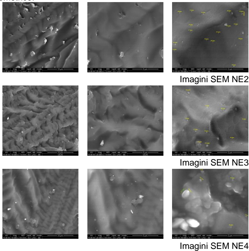
Fig. 8 Analiză SEM a materialelor NE
