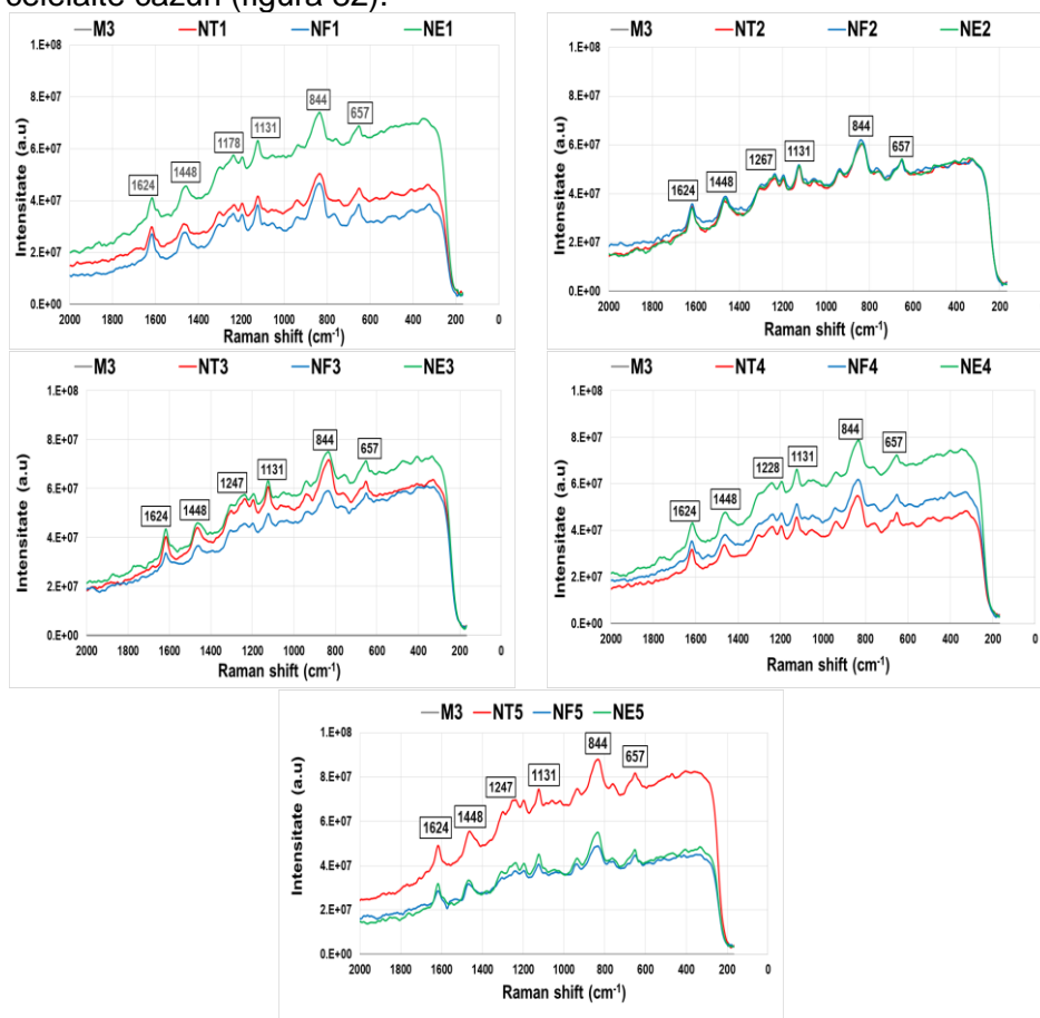
Figura 5. Spectrele Raman ale materialelor în funcție de durata menținerii tratamentului
