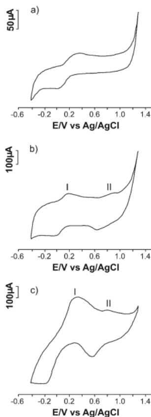
Figura VII.3. Voltamogramele ciclice ale: a) CoPc-SPCE; b) MB-SPCE; c) PB-SPCE imersați în soluție de K_4[Fe(CN)_6] 0,001 M – KCl 0,1 M înregistrate cu viteza de scanare de 0,6 \text{ V} \times \text{s}^{-1}
