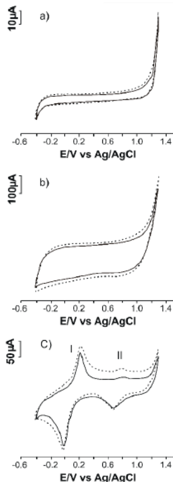
Figura VII.6. Voltamogramele ciclice ale a) CoPc-SPCE; b) MB-SPCE; c) PB-SPCE imersați în soluție de KCl 0,1 M (linia punctată) și în soluție de L-Phe 0,001 M - KCl 0,1 M (linia continuă) înregistrate cu 0,6 \text{ V} \times \text{s}^{-1}
