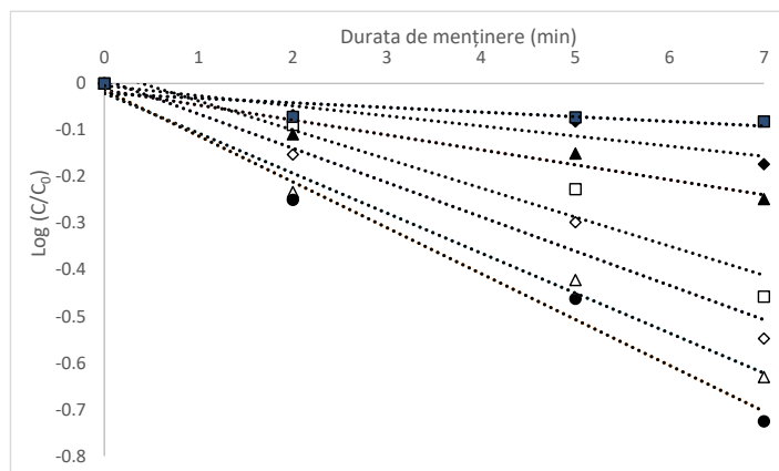
Figura 3.5. Cinetica de degradare termică a antocianilor monomerici totali în apă acidulată la pH 4.5 la temperaturi cuprinse între 120 și 180°C (■ 120°C, ◆ 130°C, ▲ 140°C, □ 150°C, ◇ 160°C, △ 170°C, ● 180°C)
